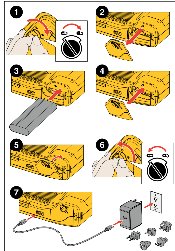
Afbeelding 1. Batterij
