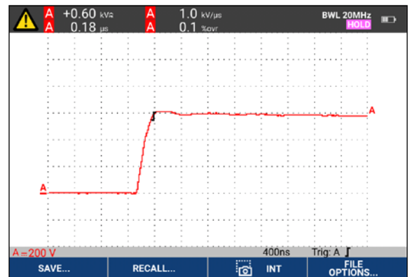
Spanningsmodulatie met zoom
