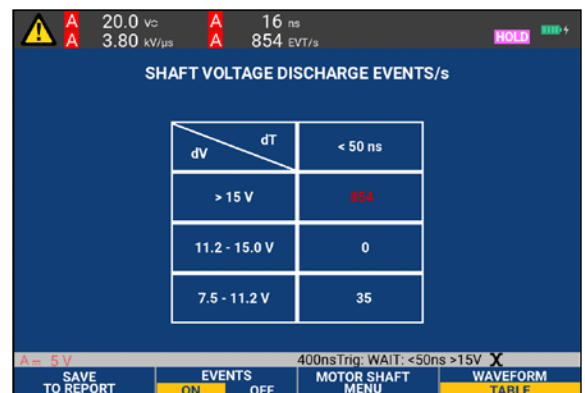
Telling van het aantal spanningsontladingen via de motoras
