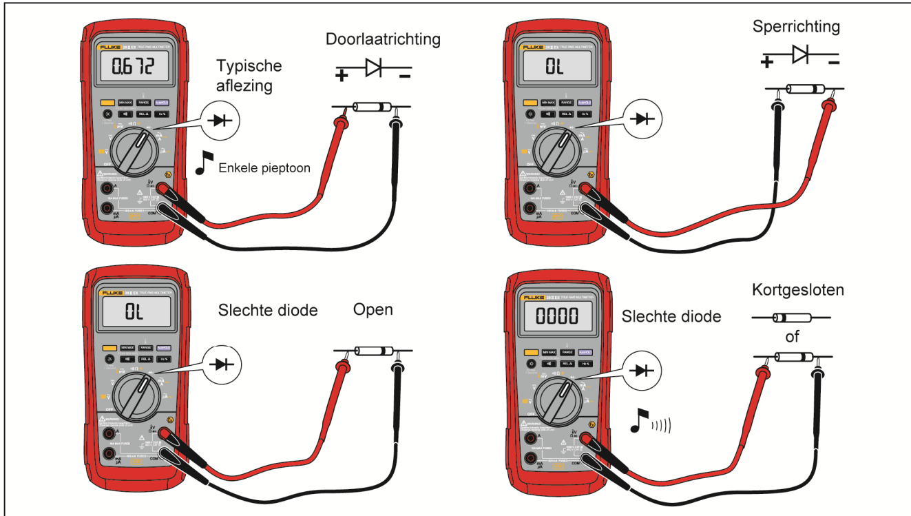
Afbeelding 7. Diodetests
