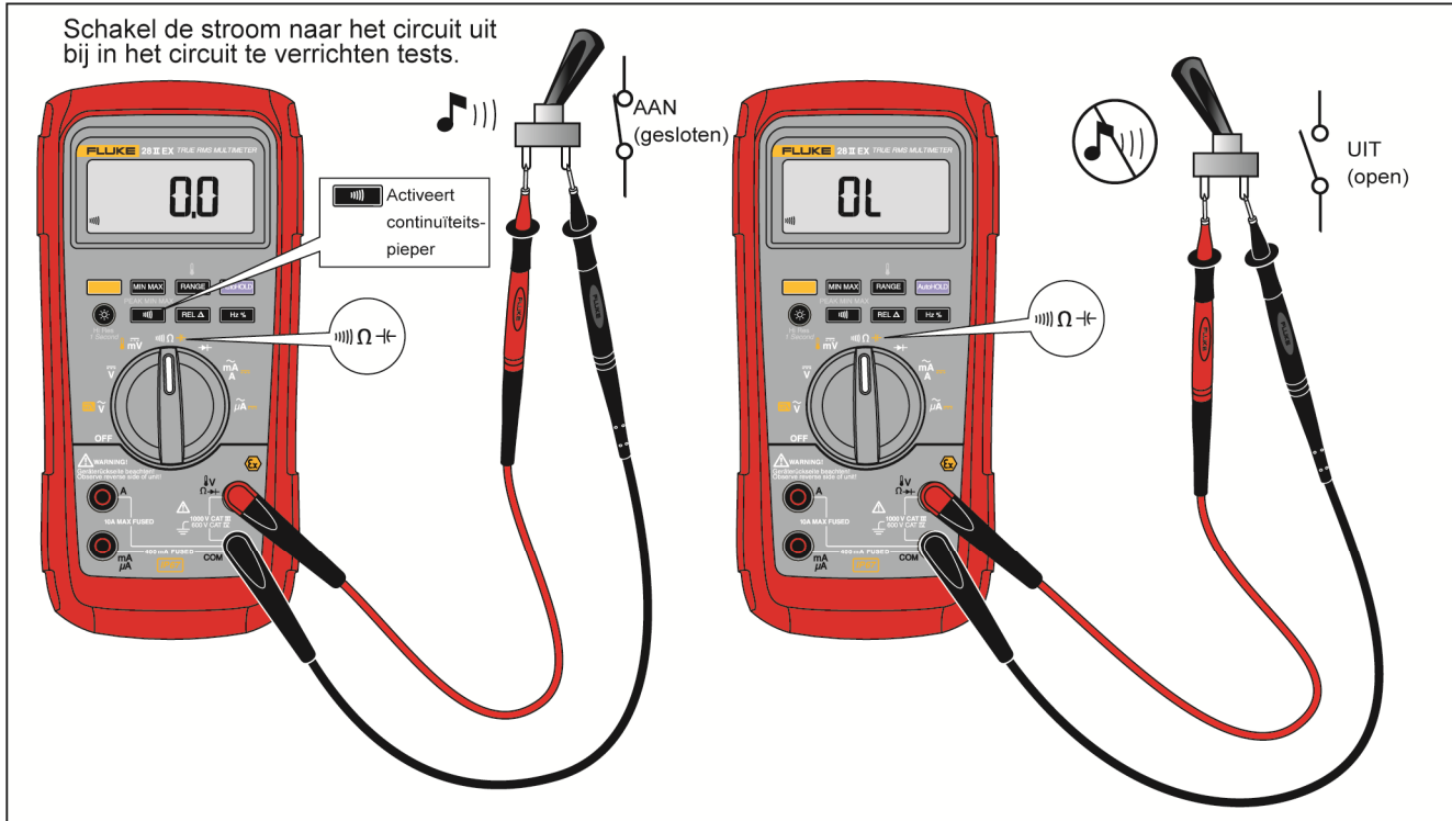
Abbeelding 4. Doorgangstests
