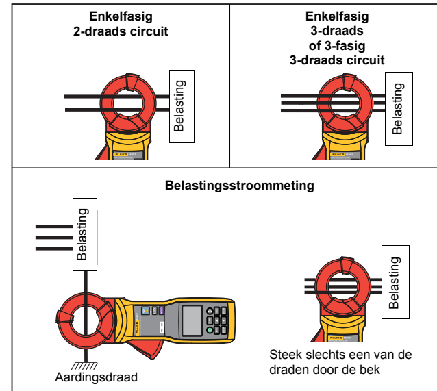
Afbeelding 9. AC-lekstrommeting
