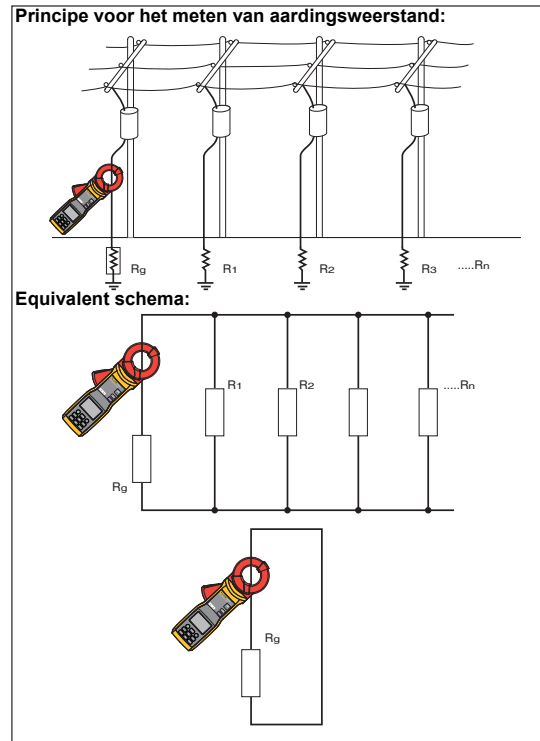
Afbeelding 8. Principes voor het meten van aardingsweerstand
