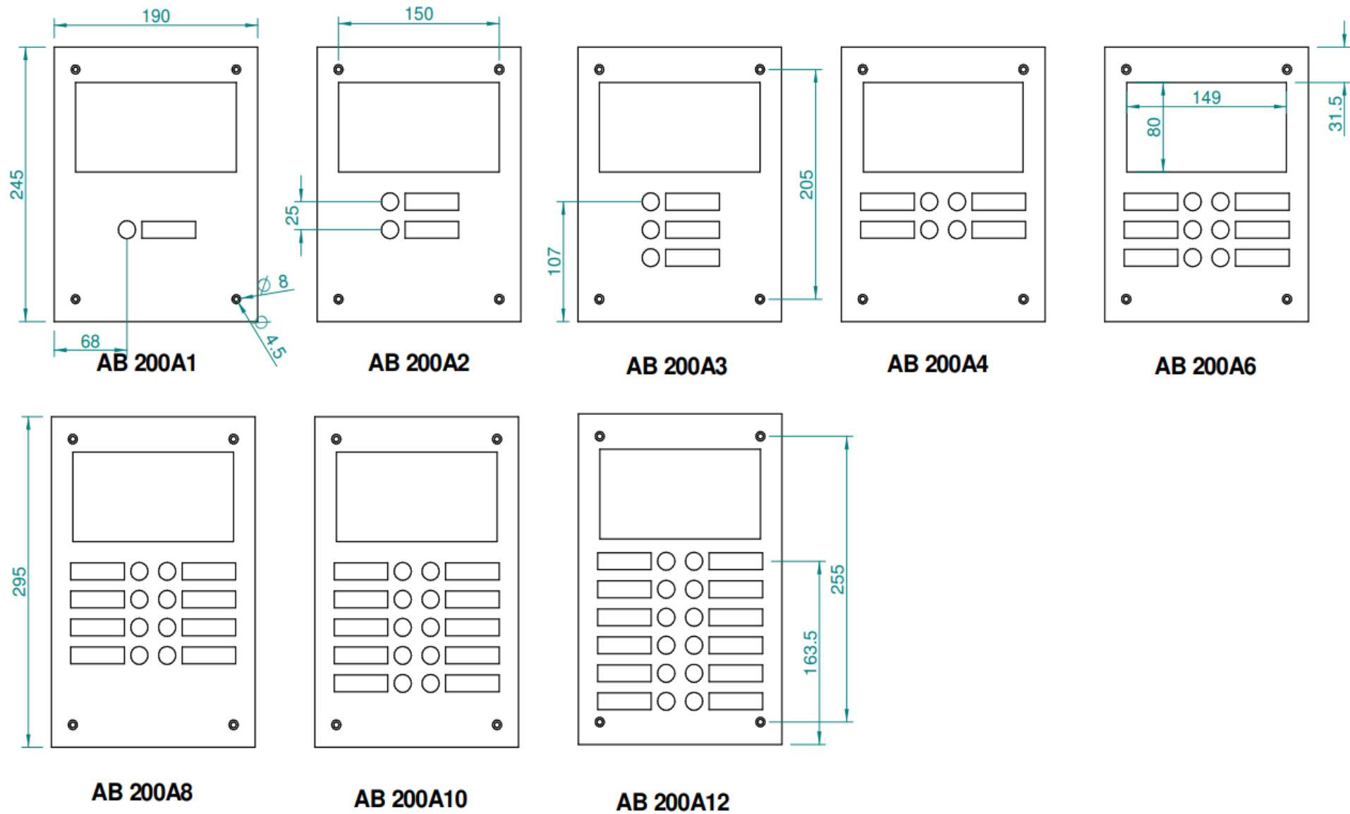
Maatvoering ATEA AB200-serie Maten in mm
